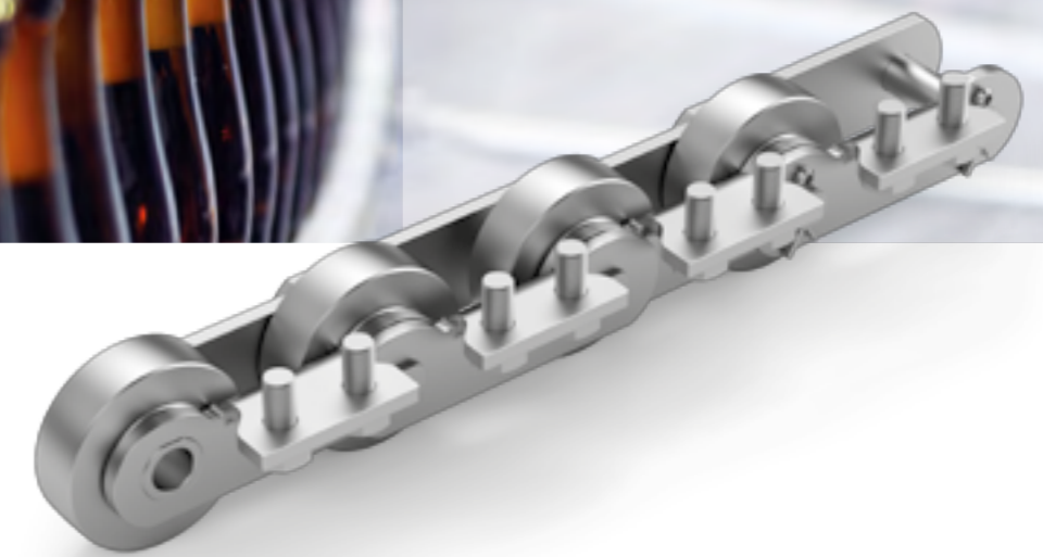
Flaschenreinigungskette mit einseitig angebogenem Winkel
